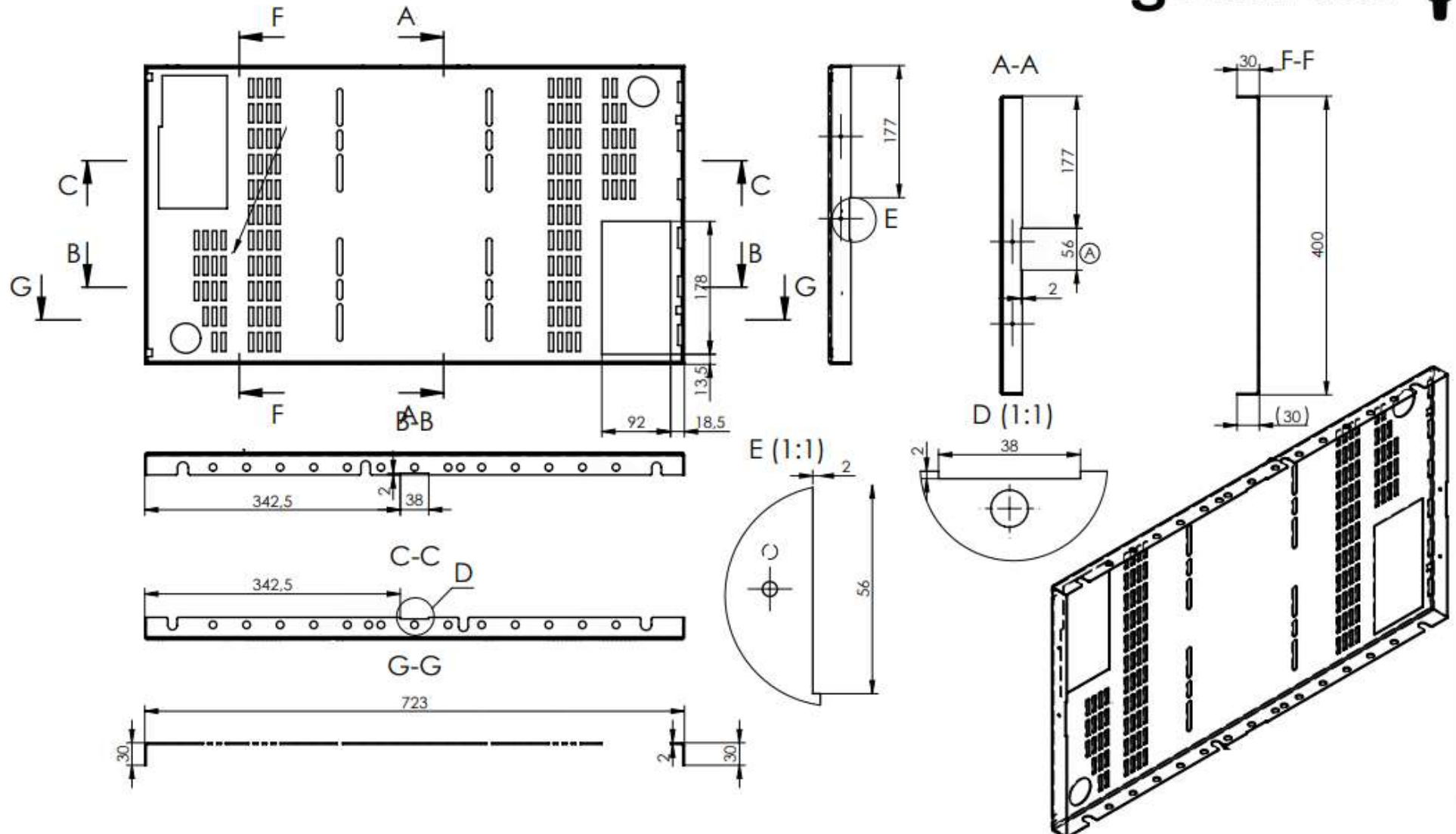
Aufputzhalterung 32" Monitorteil
