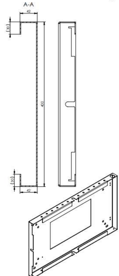
Aufputzhalterung 32" Wandteil
