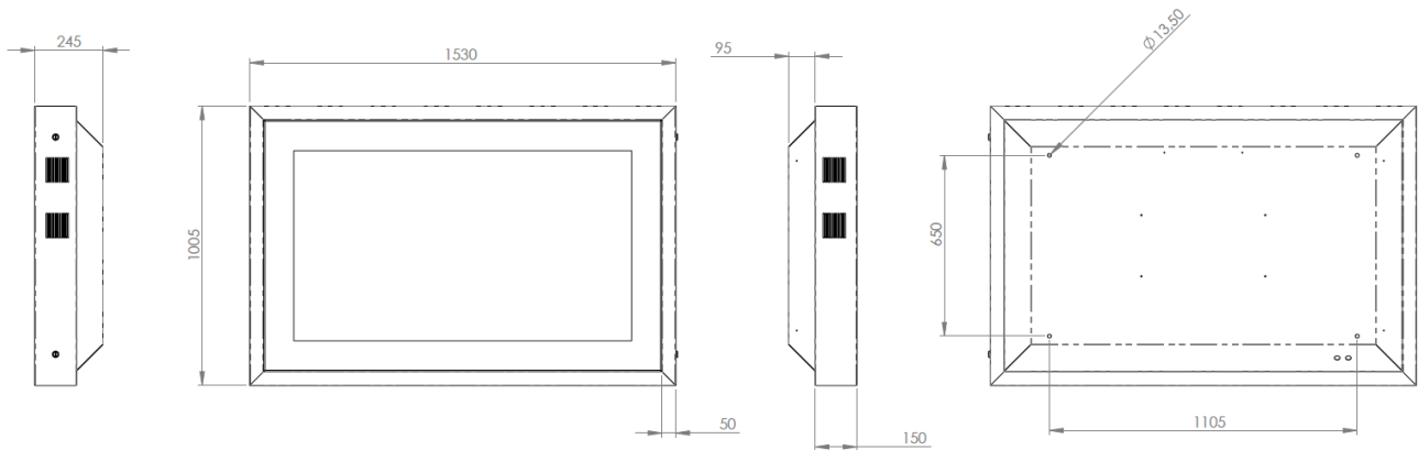
Querformat (Airtank_D_55_L) · Angaben in mm, Befestigungsbohrungen Ø 13,5 mm
