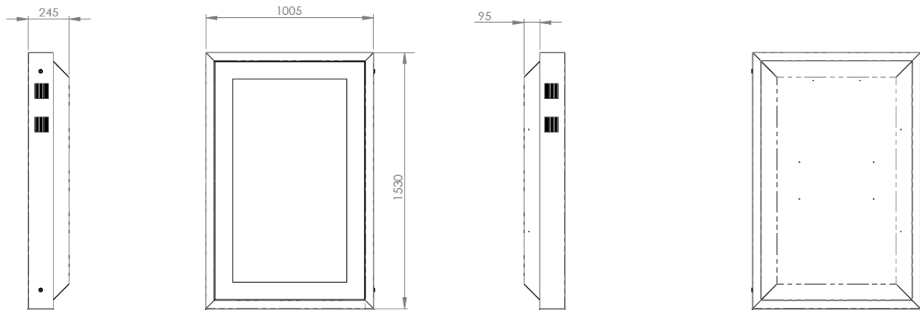
Hochformat (Airtank_D_55_P) · Angaben in mm
