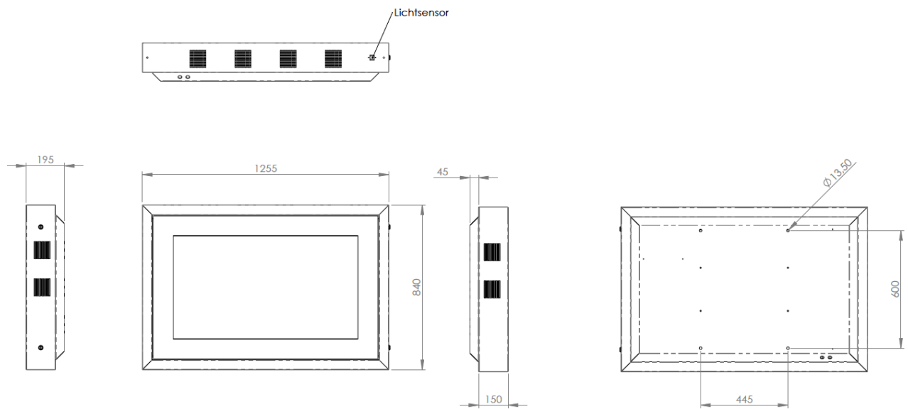
Querformat (Airtank_D_43_L) · Angaben in mm, Befestigungsbohrungen Ø 13,5 mm
