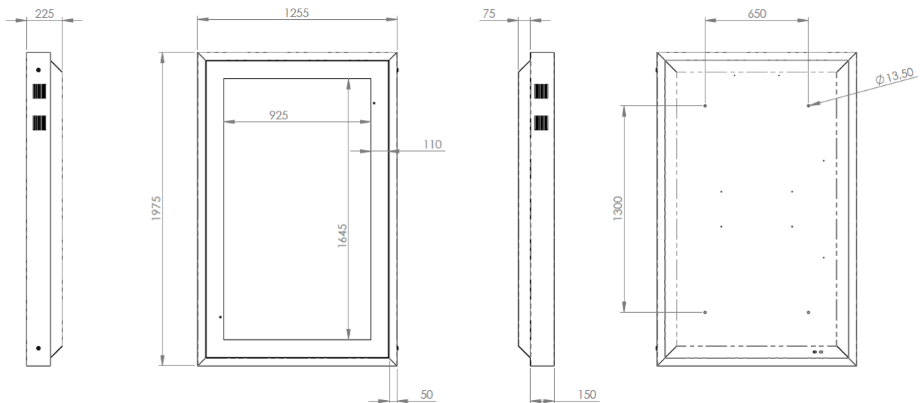
Hochformat (Airtank_D_75_P) · Angaben in mm, Befestigungsbohrungen Ø 13,5 mm
