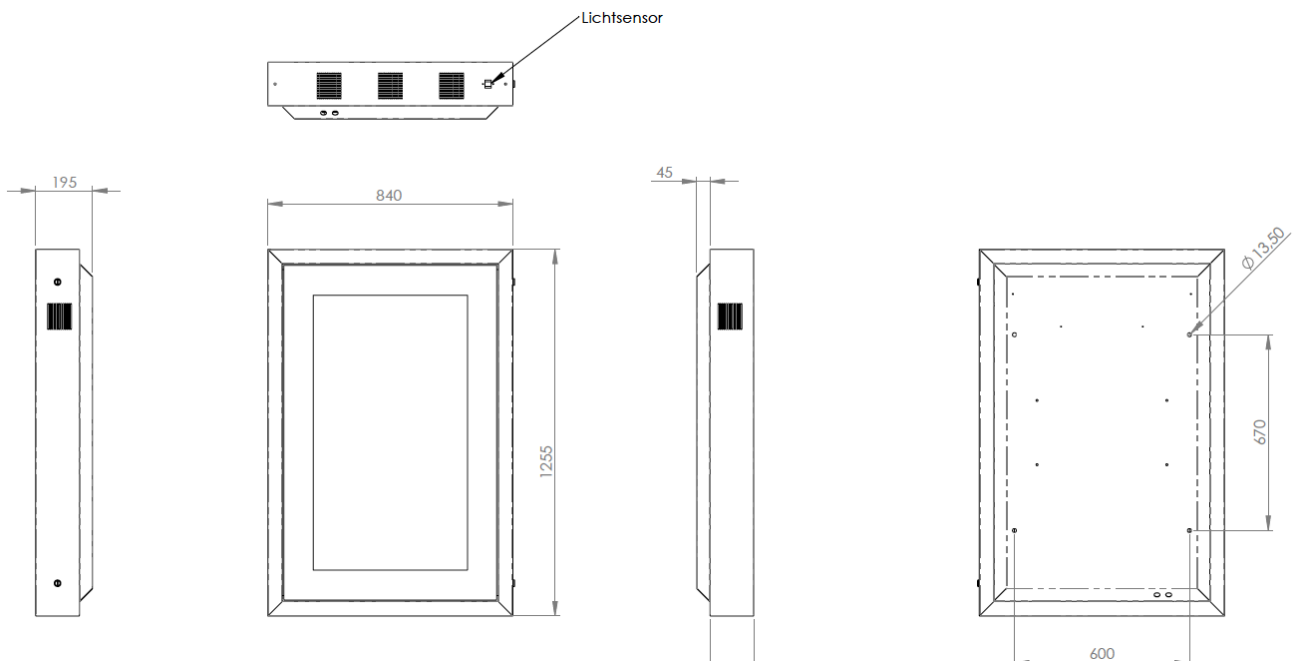
Hochformat (Airtank_D_43_P) · Angaben in mm, Befestigungsbohrungen Ø 13,5 mm
