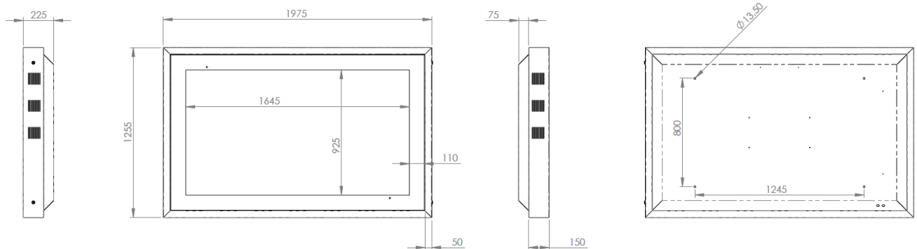
Querformat (Airtank_D_75_L) · Angaben in mm, Befestigungsbohrungen Ø 13,5 mm
